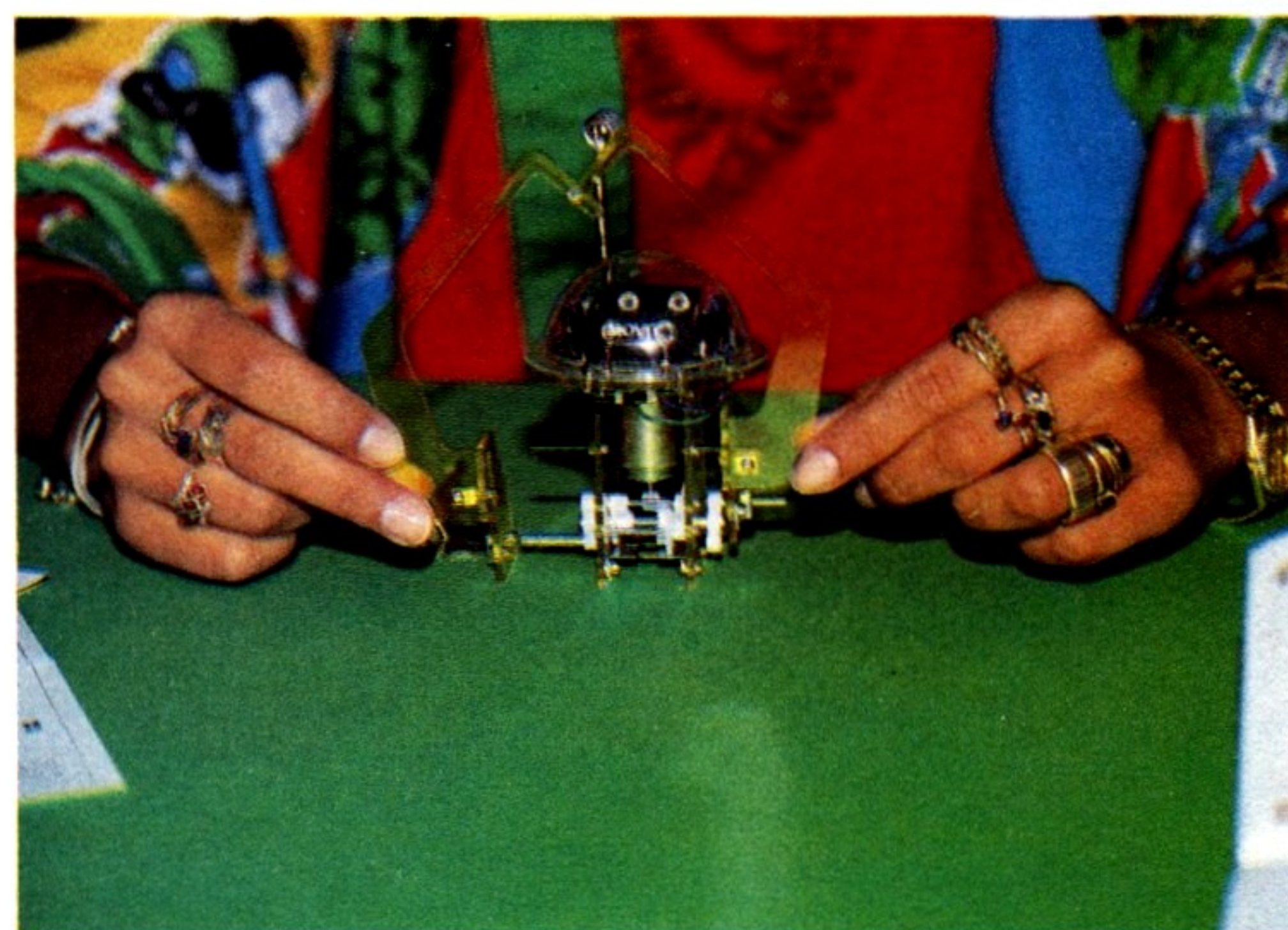
8 - Ultima fase di montaggio: si posizionano gli «arti prensili» precedentemente preassemblati, non rimane che fissarli adeguatamente.
