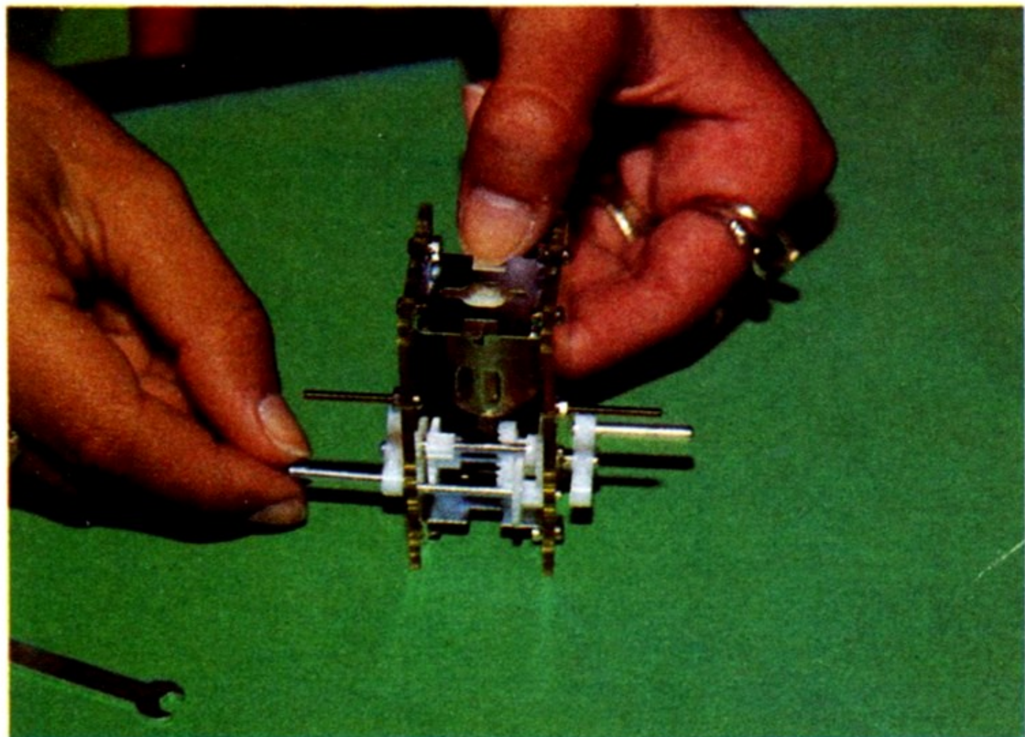
3 - Il «corpo» di Monkey è stato assemblato completamente: sono state aggiunte anche le appendici laterali che faranno da perno per il movimento delle «braccia».
