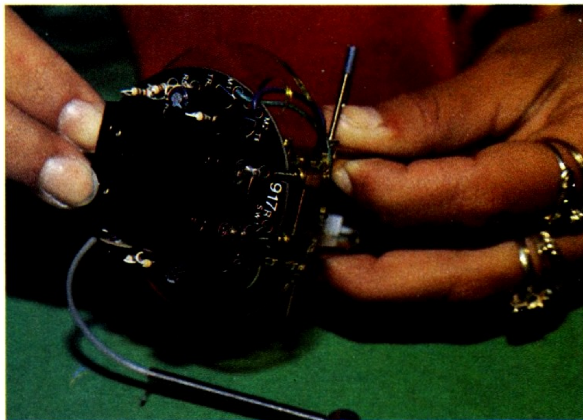
6 - Un primissimo piano del «cervello» di Monkey mentre sta per essere posizionato abilmente sui bulloni di fissaggio. Si distingue il filo schermato grigio del microfono che attiva il circuito.
