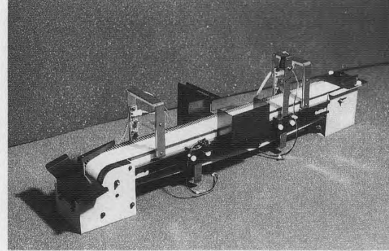
ナムコ「メカトロマスターシリーズ」のうち写真上はステップングモーター制御セット、下はシーケンス制御セット
