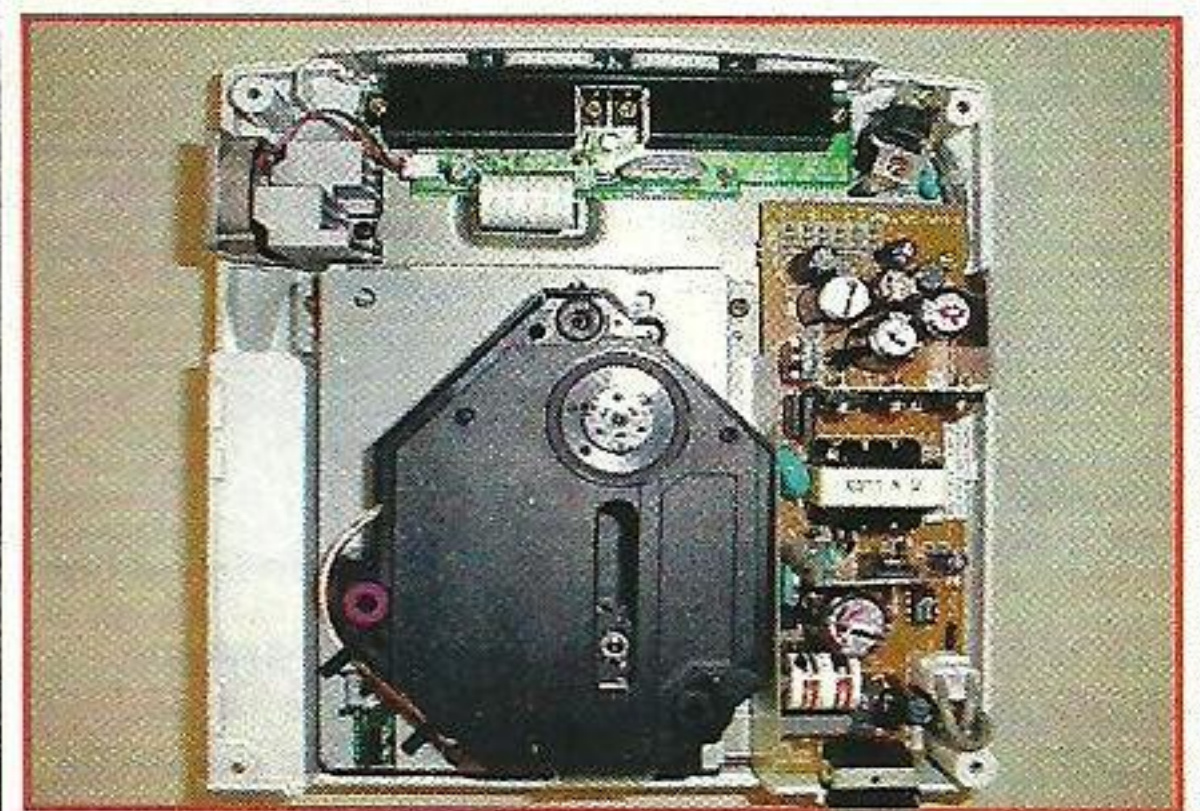
2. Dece bez obudowy. GD-ROM i zasilacz.
