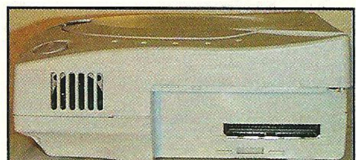
Dreamcast z boku, z wyjętym modemem - został po nim slot z piękną szyną (z prawej strony). Zwróćcie też uwagę na widoczny z lewej strony cooler - to pierwsza konsola, której procesory chłodzone są przy pomocy wiatraczka.
