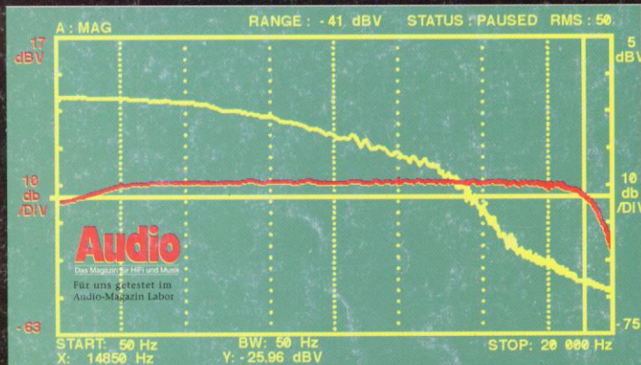
■ ATI STEREO-F/X: 44 kHz Sampling; Linearer HiFi-Frequenzverlauf ■ Herkömmliche Soundkarte: 13 kHz Sampling; fehlende Höhen, überhöhte Bässe
